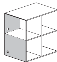
Kabelgennemføringer: udskæring i bagklædning/ korpus
